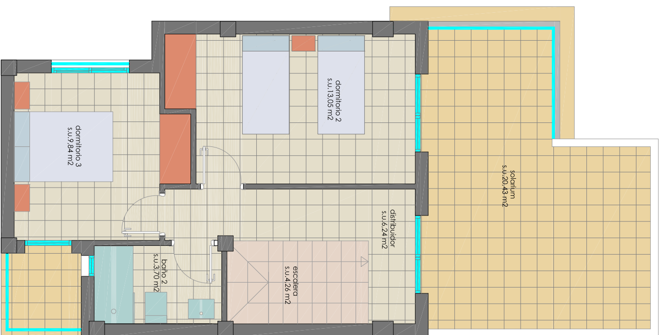
PLANTA ALTA TOP FLOOR
